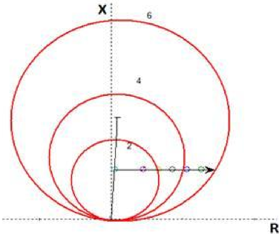
Fig. 4 Ubicación del CC en las zonas de operación del relé de distancia ubicado en la barra 1 con una resistencia de falla de 0 hasta 1,2 Ohm en el sentido de la flecha.
